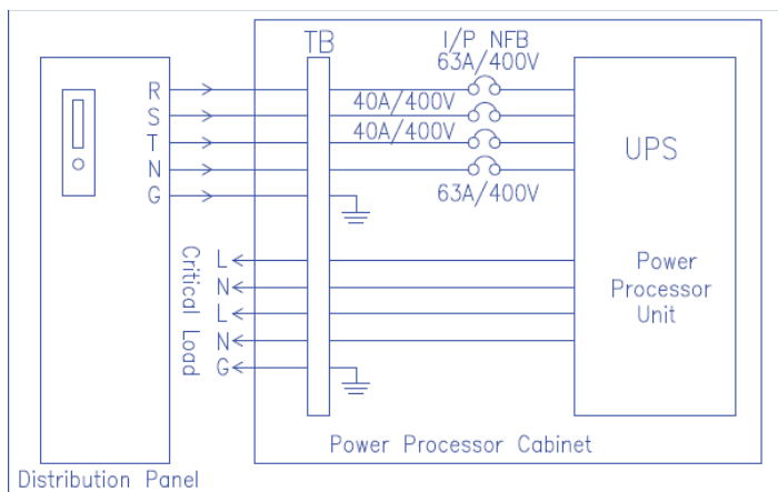
Fig b.3C-10000,3C-12000 機配線圖.
